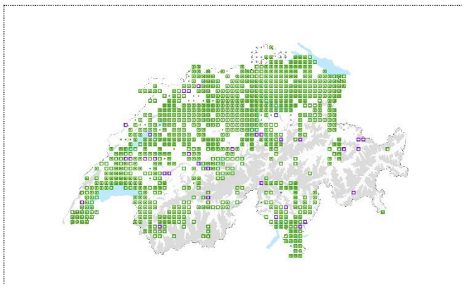
Verbreitungskarte der Reynoutria japonica (Mai 2019)
