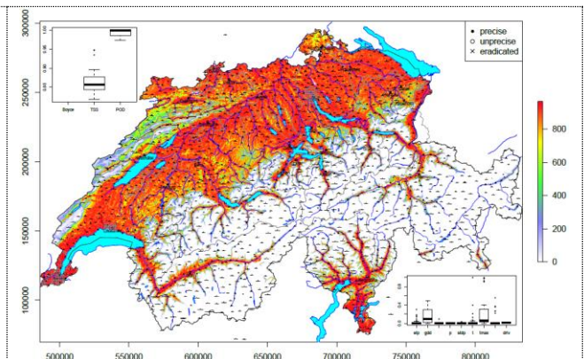
Potenzielle Ausbreitung (Modellierung UNI_Lausanne)
