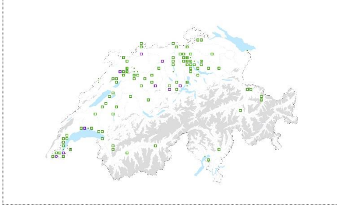
Verbreitungskarte der Reynoutria sachalinensis (Mai 2019)
